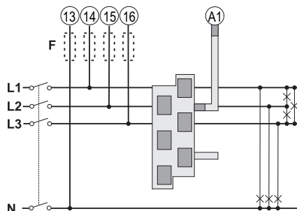
Fig. 3 Sistema trifásico, una carga trifásica.
