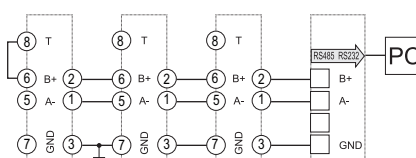
Fig. 16 Doble puerto RS485 para una conexión en cadena tipo margarita.
