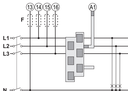
Fig. 6 Sistema trifásico, tres cargas monofásicas.
