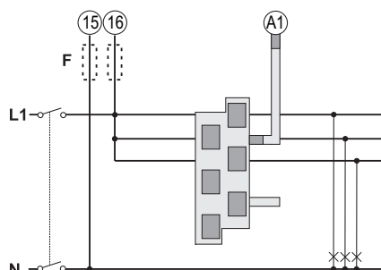
Fig. 9 Sistema monofásico, tres cargas monofásicas.
