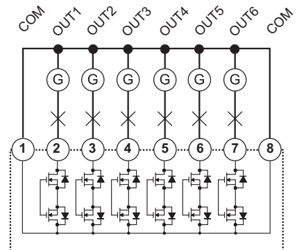
Fig. 6 M F I6 O6: salidas optomofet
