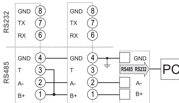
Fig. 30 M C 485232. Port série RS485.
