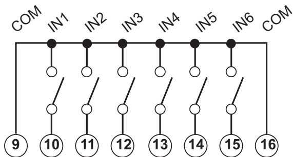
Fig. 24 MF I6 O6. 6 entrées numériques et 6 sorties statiques
