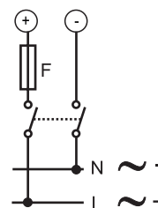
Fig. 17 Alimentation auxiliaire (H). Fusible 250 V [T] 630 mA (F). Alimentation auxiliaire (L). Fusible 250 V [T] 3,15 A (F).
