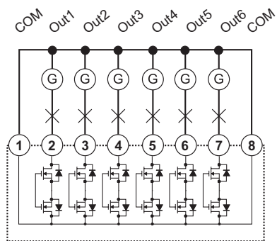
Fig. 25 MF I6 R4. 6 entrées numériques et 4 sorties relais
