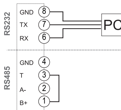
Fig. 31 M C 485232. Port série RS232.
