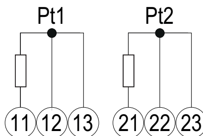
Fig. 8 Entradas de temperatura 1 y 2 (3 cables)
