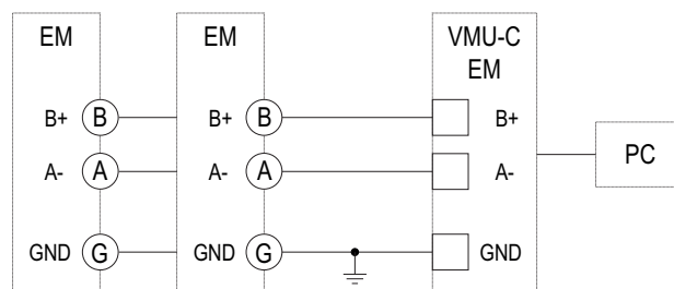
Fig. 2 RS485 COM2 a los medidores de energía
