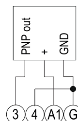
Fig. 16 Entrada de pulso PNP (código del producto: 2TIW)
