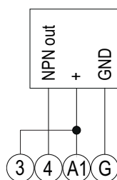
Fig. 15 Entrada de pulso NPN (código del producto: 2TIW)
