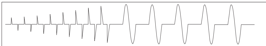
Démarrage progressif avec ON/OFF, Burst, Distributed full cycle et Advanced full cycle.
