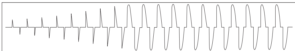
Démarrage progressif avec angle de phase
