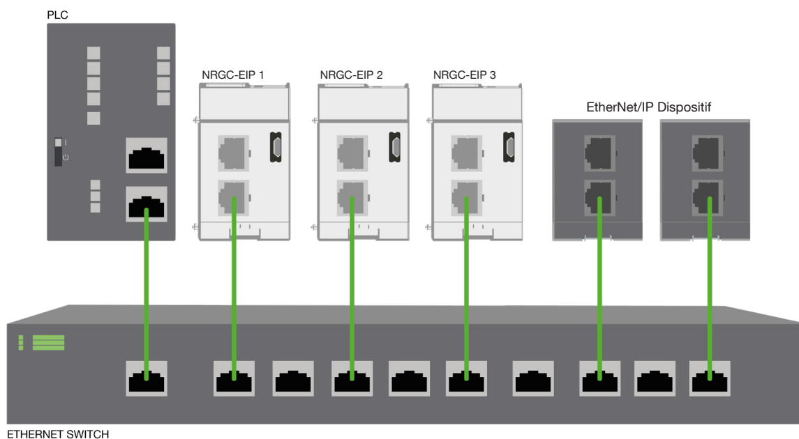
Fig. 4 Exemple d'une configuration en étoile du NRGC-EIP avec d'autres appareils et contrôleur EtherNet/IP
