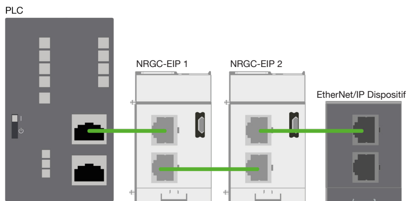
Fig. 3 Exemple d'une configuration en ligne du NRGC-EIP avec d'autres appareils et contrôleur EtherNet/IP
