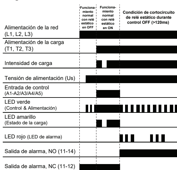
Diagrama de funcionamiento 5:
