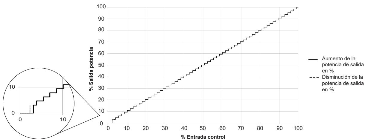
Modo de conmutación de 4 ciclos completos: RGC...C4
