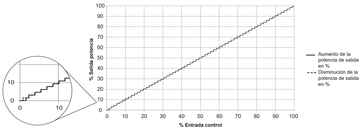
Modo de conmutación de 1 ciclo completo: RGC...C1
