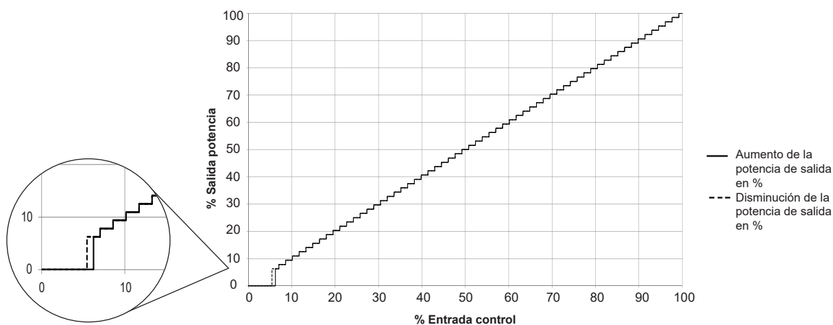
Modo de conmutación de 16 ciclos completos: RGC...C16
