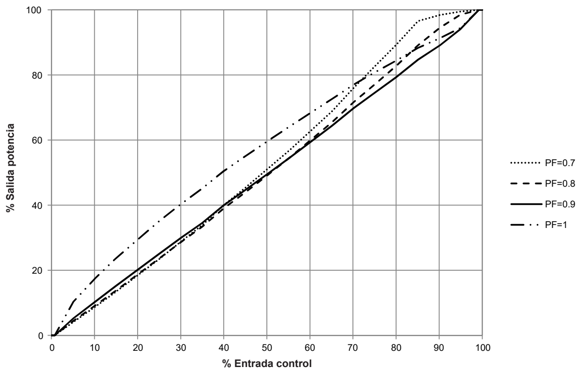
3 fases, sistemas de 4 hilos
