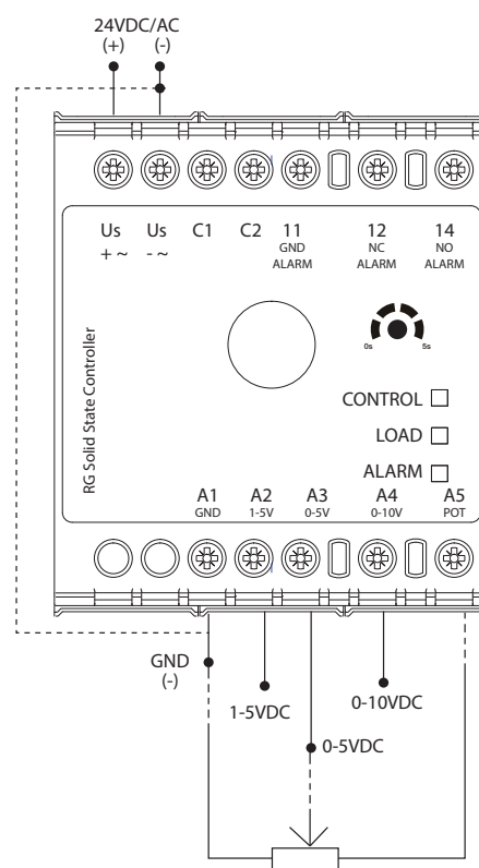
Entrada tipo 'S16', alimentación externa CC RGC..V..S16
