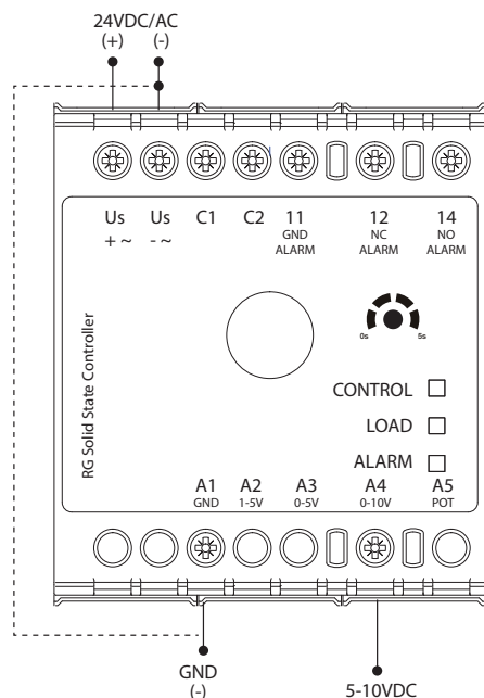
Entrada tipo 'S', alimentación externa CC RGC..V..S
