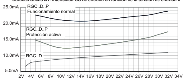
Características A1: Intensidad CC de entrada en función de la tensión de entrada x
