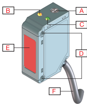
Fig. 1 Câble
