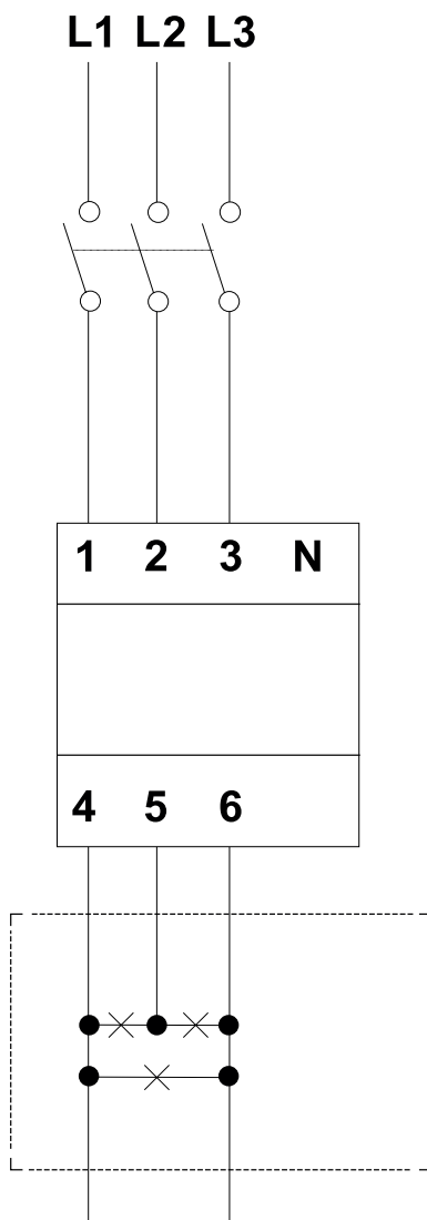
Triphasé sans neutre (3 fils)
