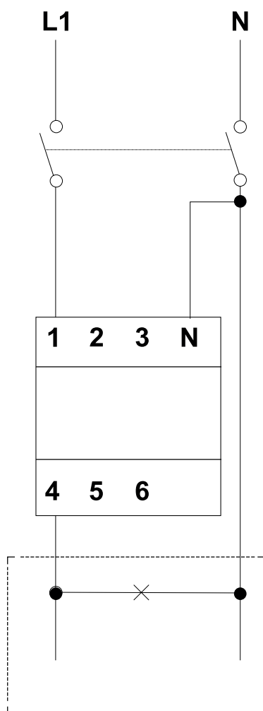
Système monophasé.
