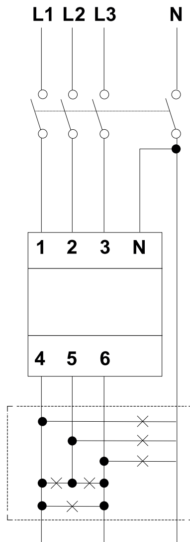
Triphasé avec neutre (4 fils).
