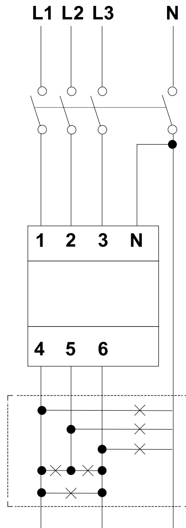
Trifásico con neutro (4 hilos)
