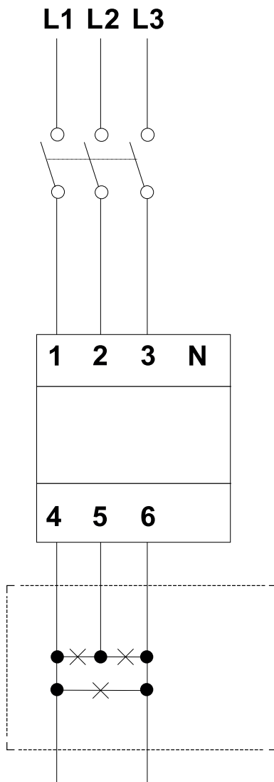
Trifásico sin neutro (3 hilos)
