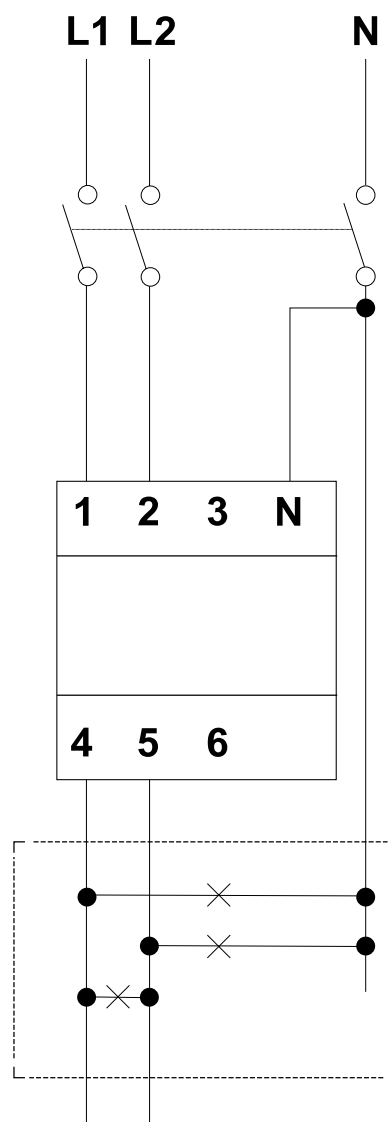
Sistema bifásico
