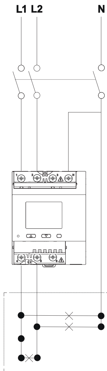
Fig. 6 Biphasé (3 fils)
