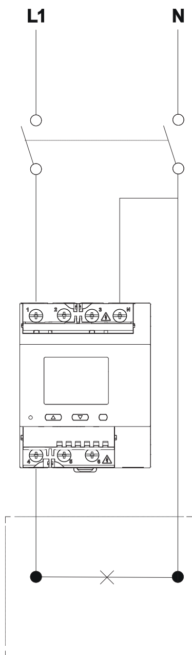
Fig. 5 Système monophasé.
