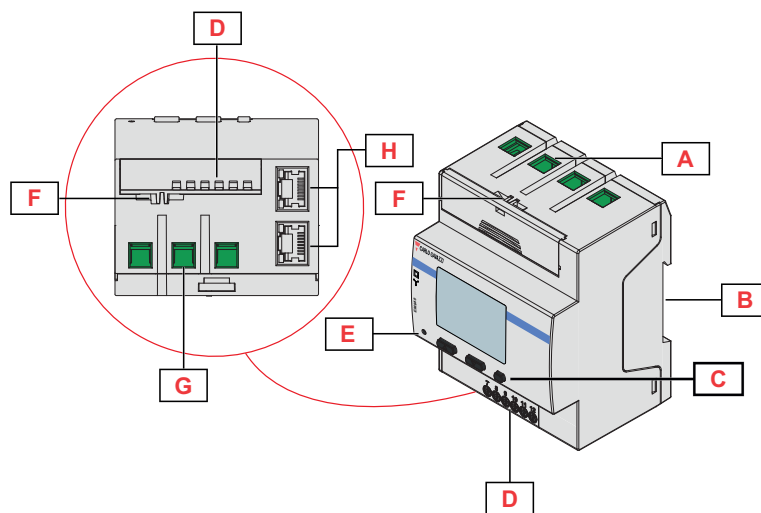
Fig. 1 EM640 Devant
