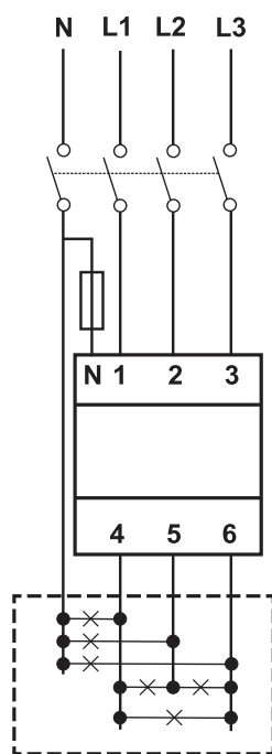
Fig. 3 Triphasé sans neutre (4 fils)
