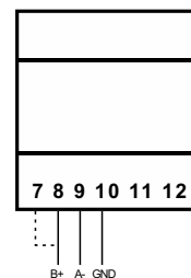
Fig. 10 Dernier appareil sur RS485
