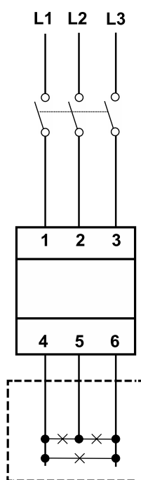
Fig. 4 Triphasé sans neutre (3 fils) MID
