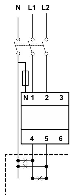
Fig. 5 Système biphasé avec neutre (3 fils).
