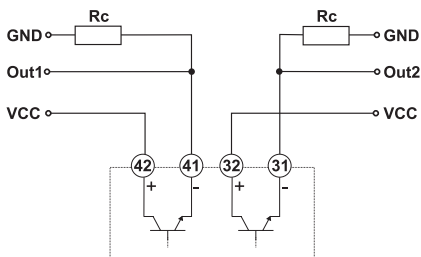
Fig. 26 Salidas estáticas, referencia VCC
