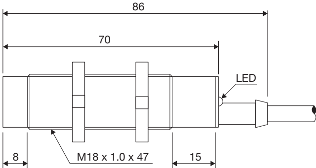
Fig. 7 Cable CA18CAN...A2IO
