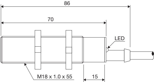
Fig. 6 Cable CA18CAF...A2IO
