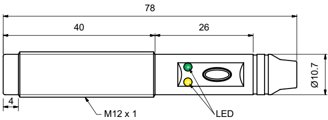
Fig. 7 Cable CA18EAN...A2IO
