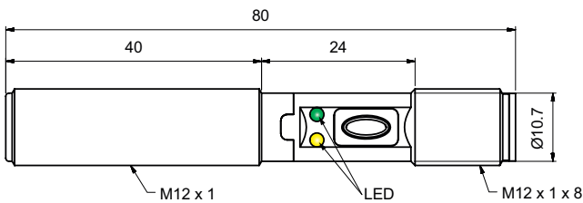
Fig. 8 Conector CA18EAF...M1IO
