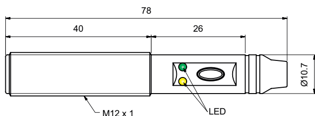
Fig. 6 Cable CA18CAF...A2IO
