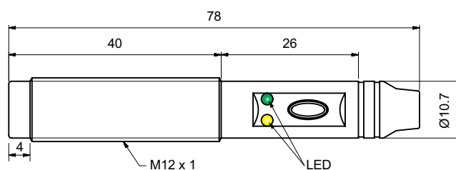
Fig. 7 Cable CA18CAN...A2IO
